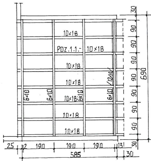
RZUT KONSTR. DACHU
