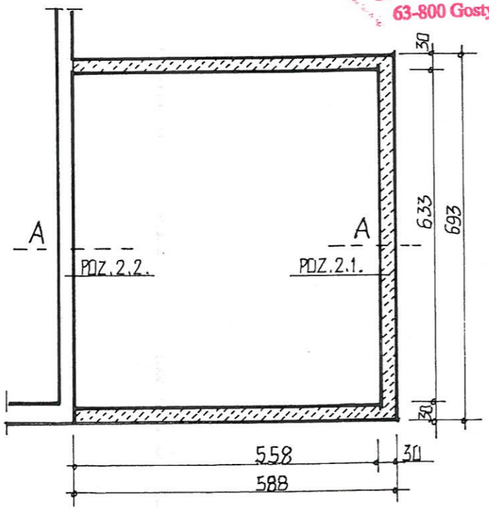
RZUT FUNDAMENTÓW
