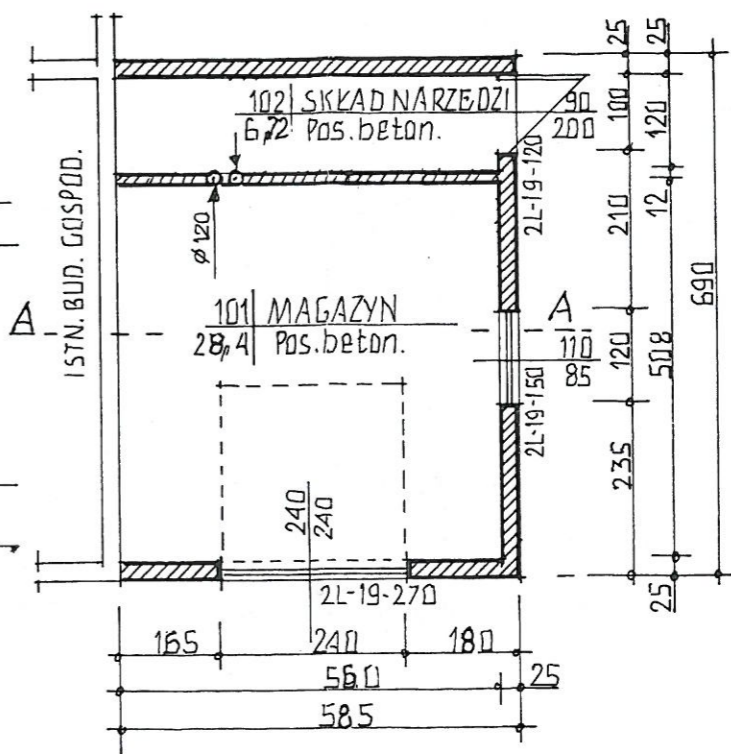
RZUT PRZYZIEMIA
