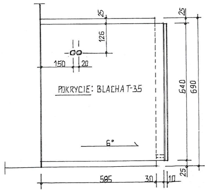
RZUT POŁĄCZ DACHOWEJ
