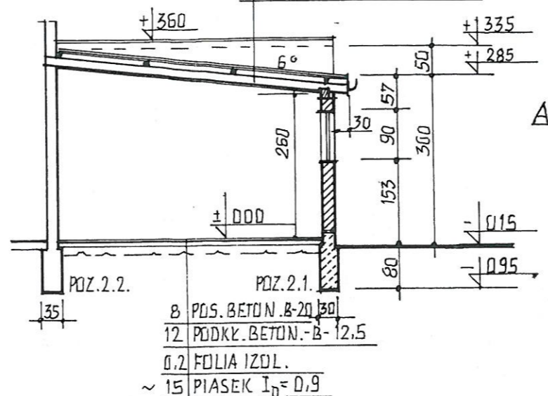
PRZEKRÓJ A-A
